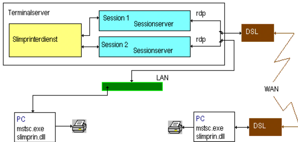
Komponentenübersicht Slimprinter
